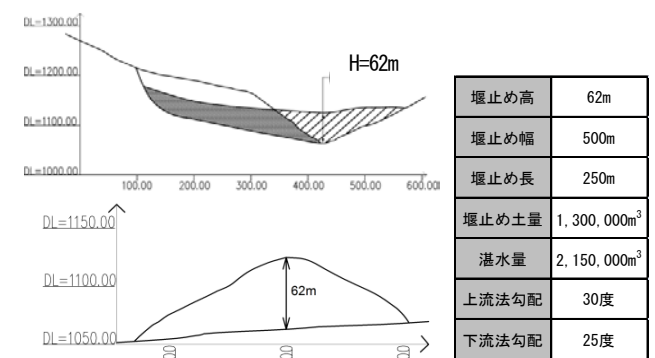
図 3 河道閉塞の形状（上：横断面 下：縦断面）
