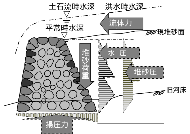
図-1 満砂時の荷重条件概念
