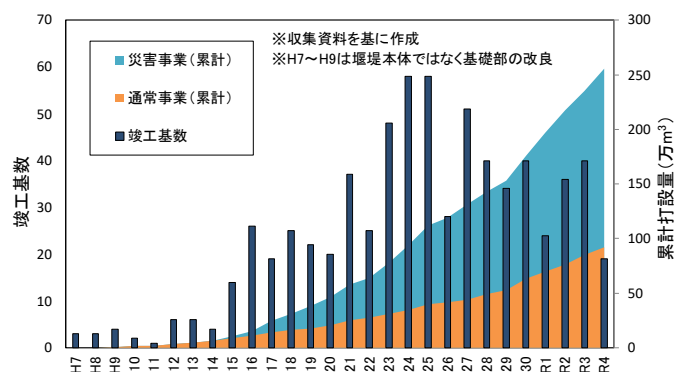
図-1 砂防ソイルセメント堰堤基数及び打設量推移
