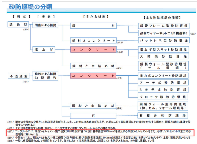
図-2 砂防堰堤の分類
